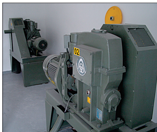
Figura 79: Casa de máquinas dos elevadores
