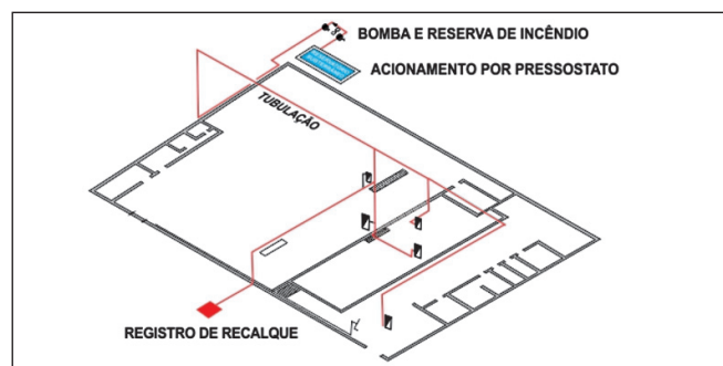
Figura 65: Perspectiva isométrica de sistema de hidrantes
