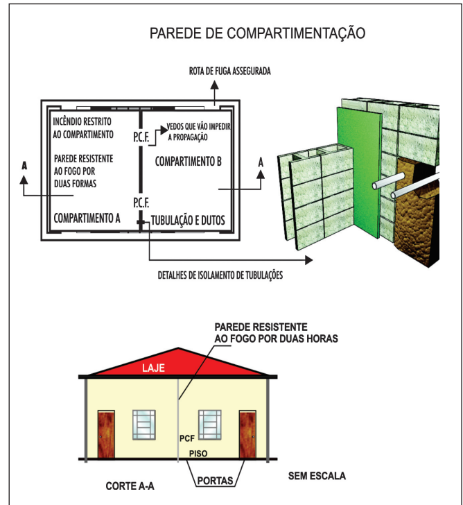
Figura 32: Detalhes de parede de compartimentação
