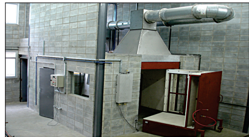
Figura 43: Reação do fogo em materiais de construção
